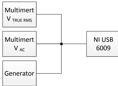
Rys.1. Układ pomiarowy pomiarowy
